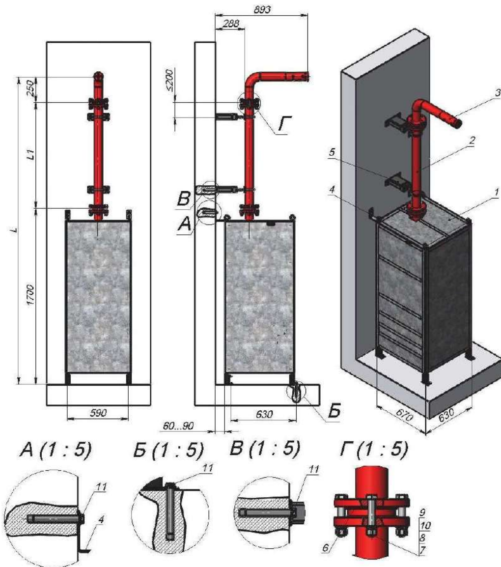
Рисунок П.2.1 Монтаж модуля с верхним выходом. Вертикальное удлинение трубопровода подачи ГПОВ.
