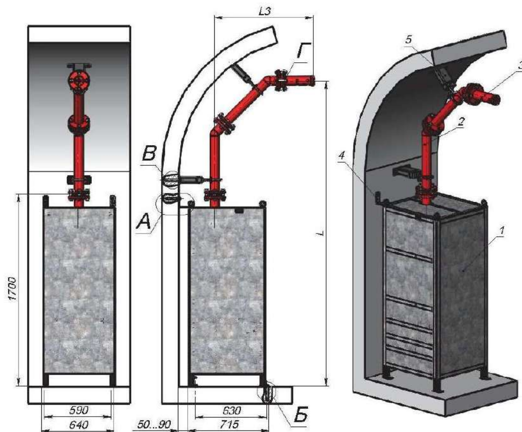
Рисунок П.2.5 Монтаж модуля с верхним выходом. Удлинение трубопровода подачи ГПОВ помещениях со сферическим потолком.
