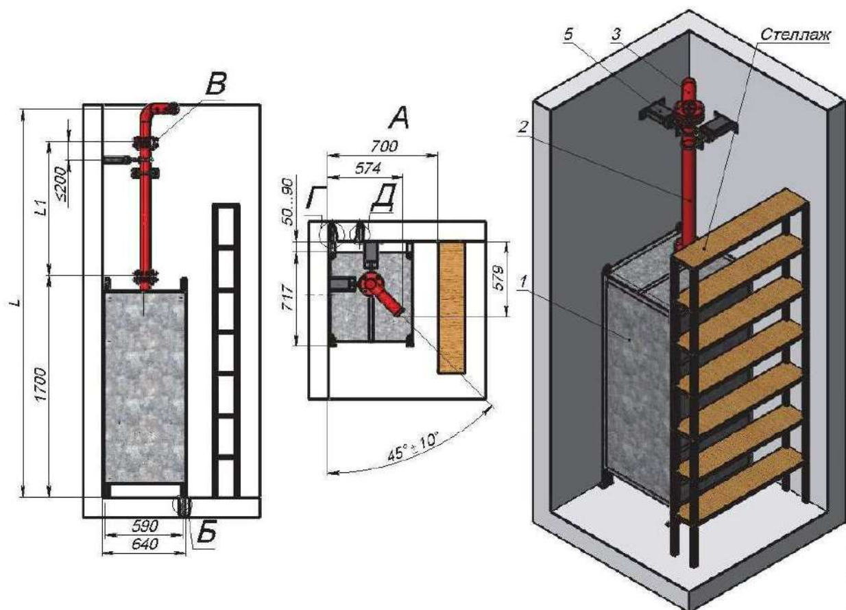
Рис П2.6 Монтаж модуля с верхним выходом при монтаже в углу.
