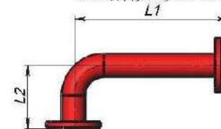
Рисунок П.2.3 Монтаж модуля с верхним выходом. Вывод трубопровода подачи ГПОВ через стену.
