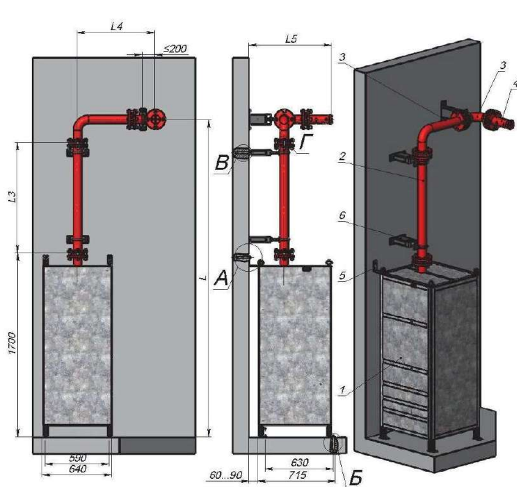
Рисунок П.2.3 Монтаж модуля с верхним выходом. Вывод трубопровода подачи ГПОВ через стену.
